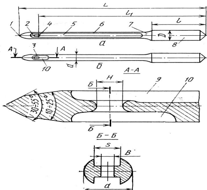
Сурет 1 - Түзі тігін машинасының инесі мен көзі
