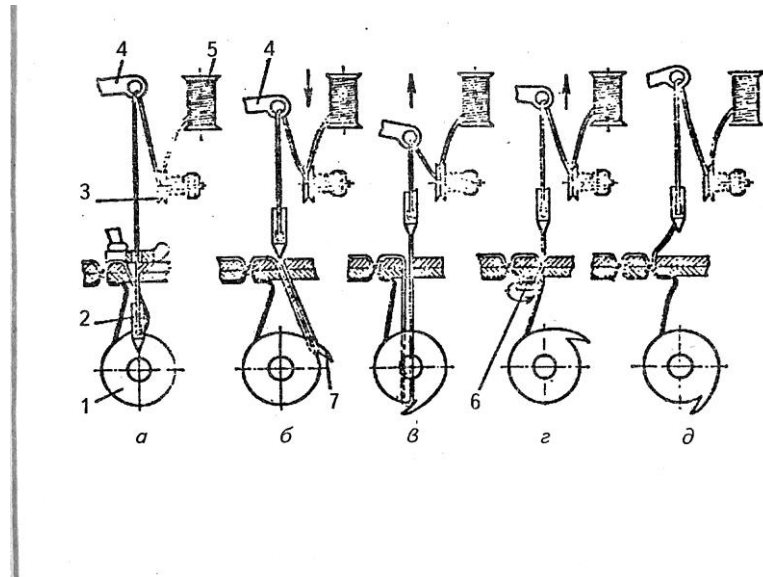
Сурет 4 - Қайық тігісінің пайда болу принципі: 1- қайық; 2-ине; 3-жіп реттегіш табақша; 4- жіптартқыш; 5-тиек немесе бобина; 6- тісті рейка.
