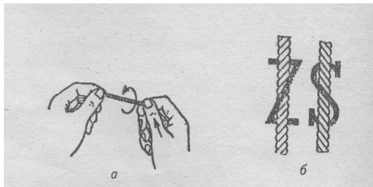
Сурет 2 - Жіптің шыйратылуы: а –жіптің шыйратылуын анықтау; б - оңға және солға шыйратылуы.
